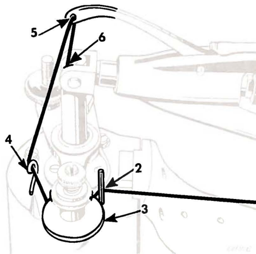
Fig. 20. Upper Threading
